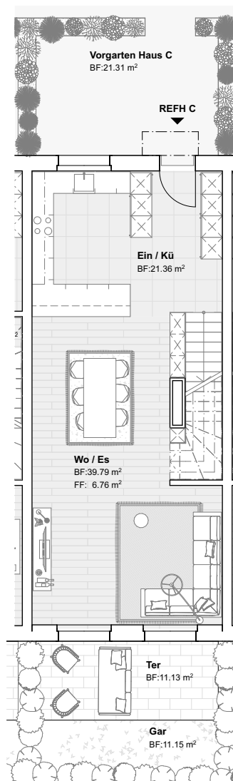
Erdgeschoss
